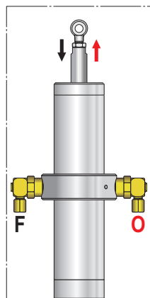
Vérin fourni avec 2 raccords tournants
