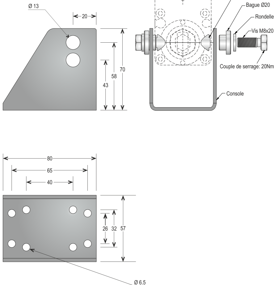
Console fournie avec son dispositif de fixation
